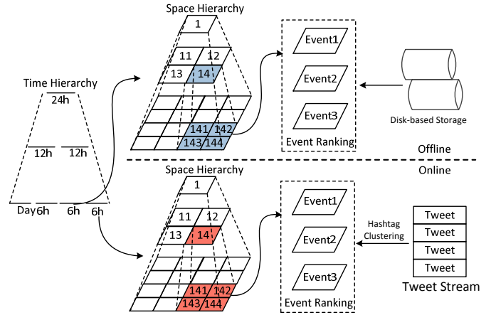
Fig. 2. Framework
